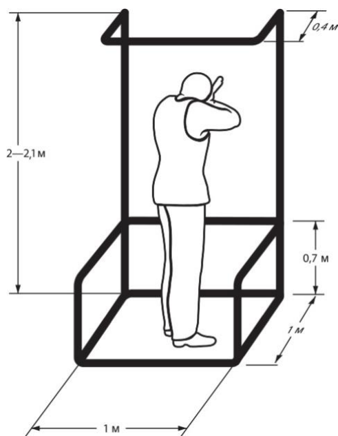
Рисунок 2-1. Устройство стрелкового места для «спортинг-компакта».
